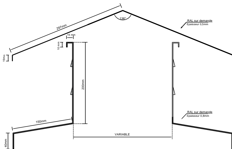
FAITAGE VENTILÉ
