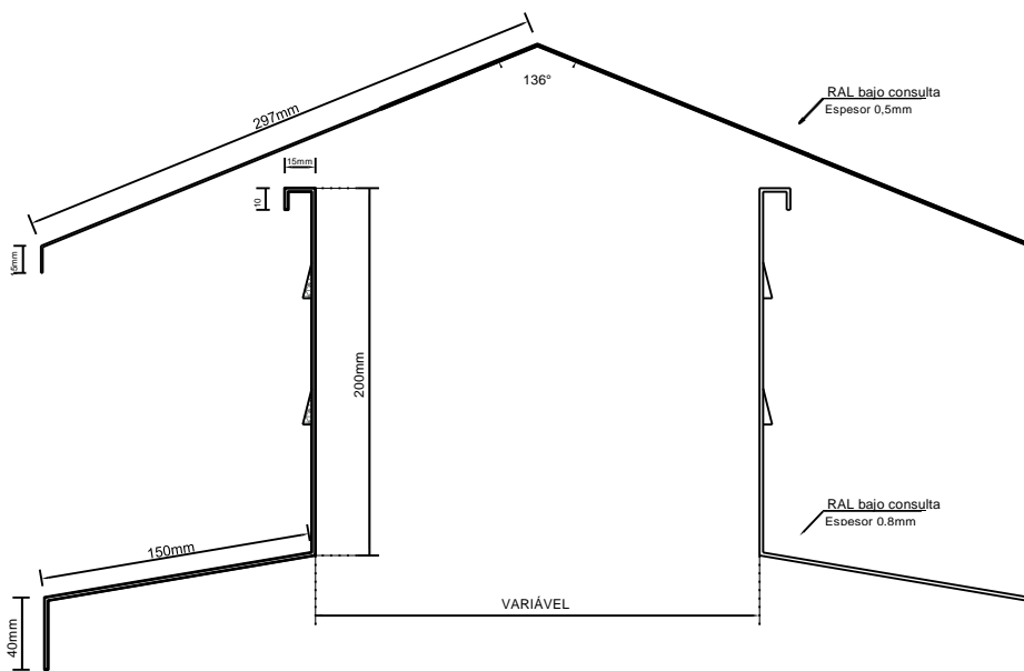
CUMBRERA VENTILADA
