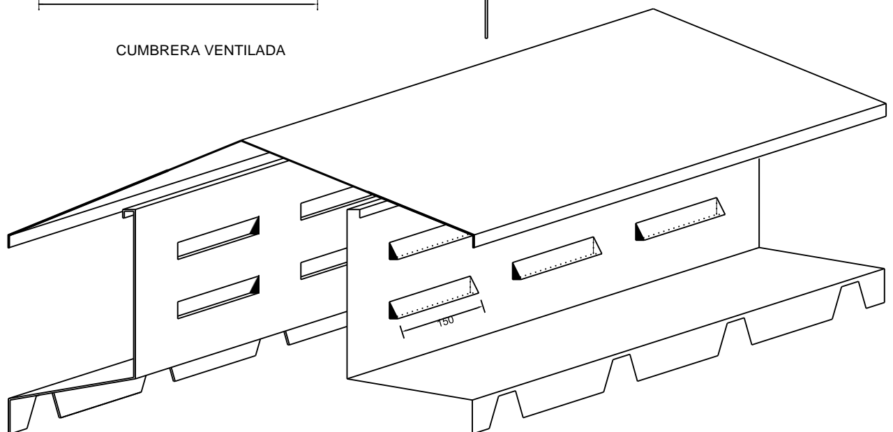
VISTA 3D DE CUMBRERA VENTILADA
